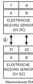
Klemmleiste 1 (Im Backupheizer)
