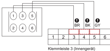
Klemmleiste 3 (Innengerät)
