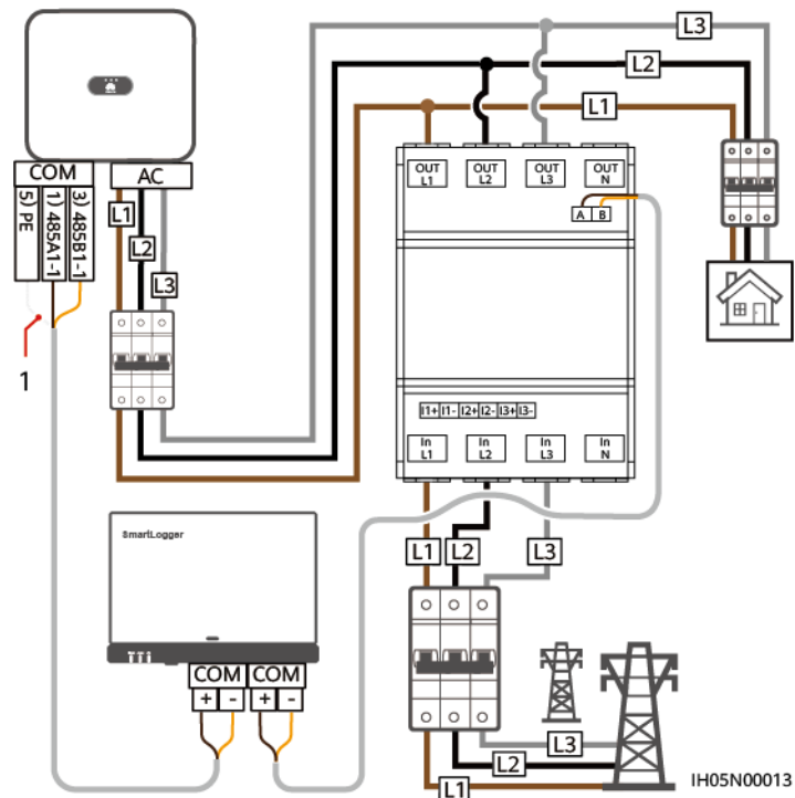
Abbildung 5-28 Dreiphasige dreiadrige Direktverbindung (SmartLogger-Vernetzung)
