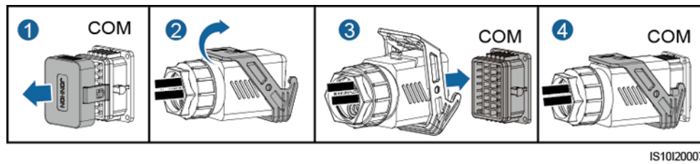
Abbildung 5-33 Sichern des Signalkabelsteckverbinders
