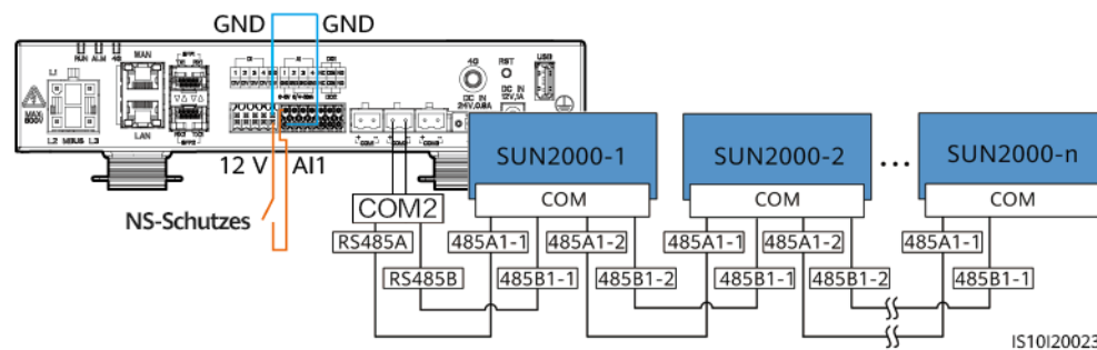
Abbildung 5-48 Anschließen des SmartLoggers an den NS-Schutzschalter
