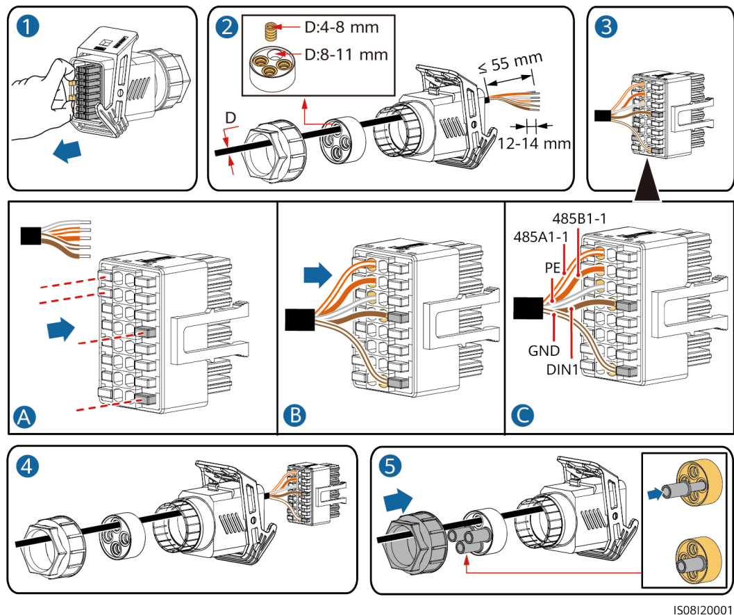
Abbildung 5-38 Kabelmontage
