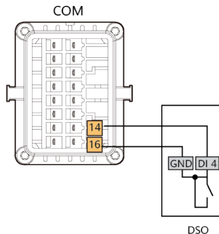
Abbildung 7-5 Kabelverbindungen
