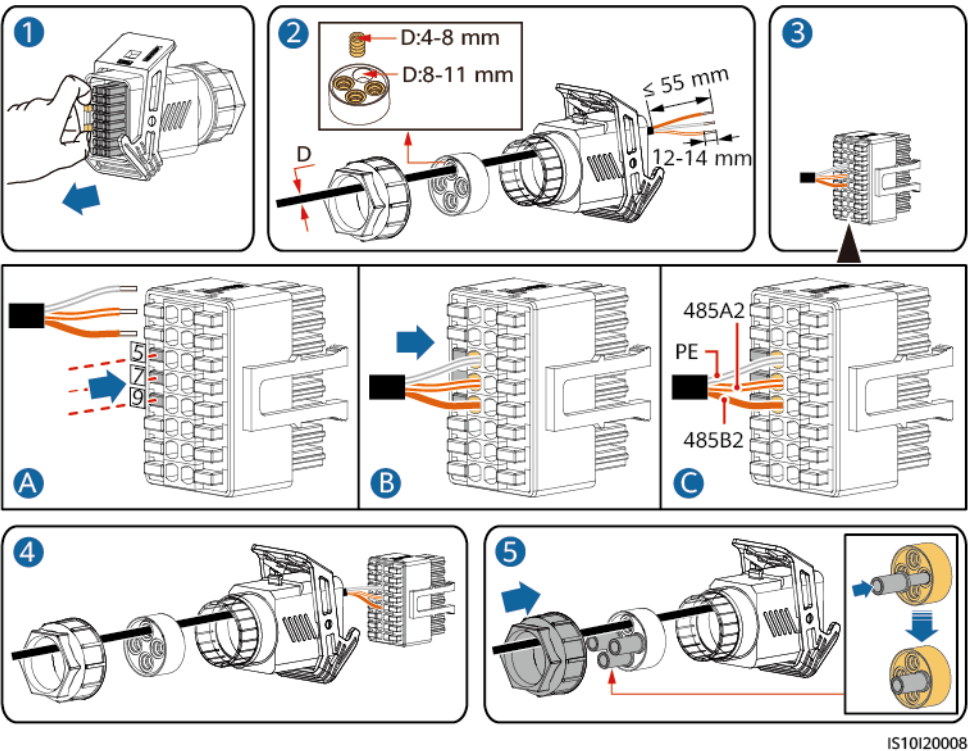
Abbildung 5-30 Kabelmontage
