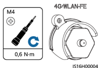
Abbildung 5-52 Installation der Anti-Diebstahl-Komponenten für den Smart Dongle
