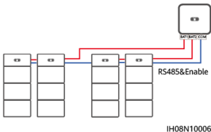
Abbildung 2-8 Anschluss des Wechselrichters an vier Batterien
