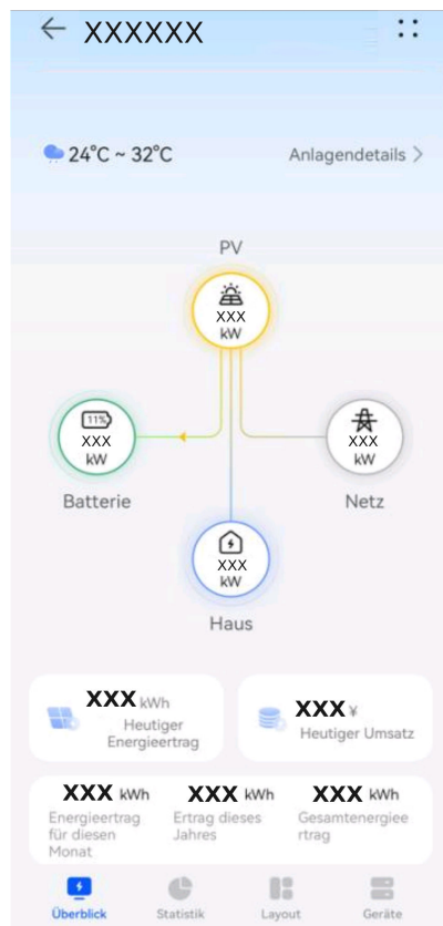
Abbildung 7-10 Anzeige des Erstellungsstatus der Anlage
