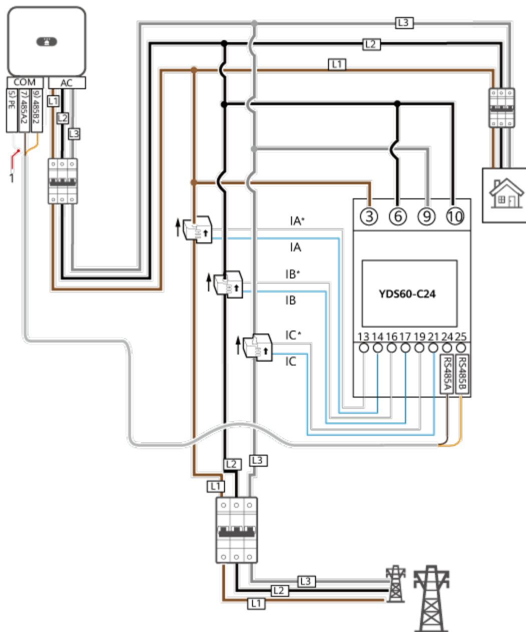
Abbildung 5-24 YDS60-C24 dreiphasige dreiadrige Kabelverbindung (Smart Dongle-Vernetzung)
