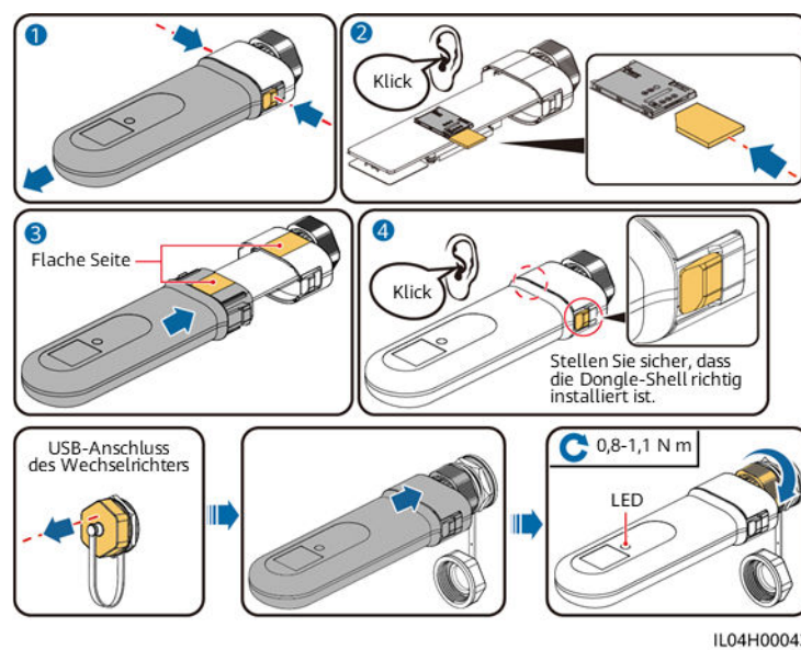
Abbildung 5-51 Installieren von 4G Smart Dongle (SDongleB-06)
