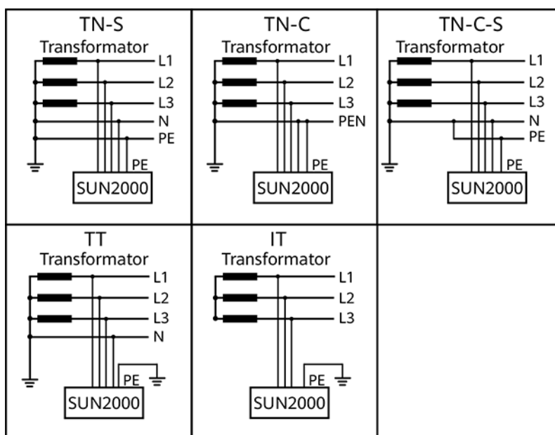
Abbildung 2-9 Unterstützte Stromnetze
