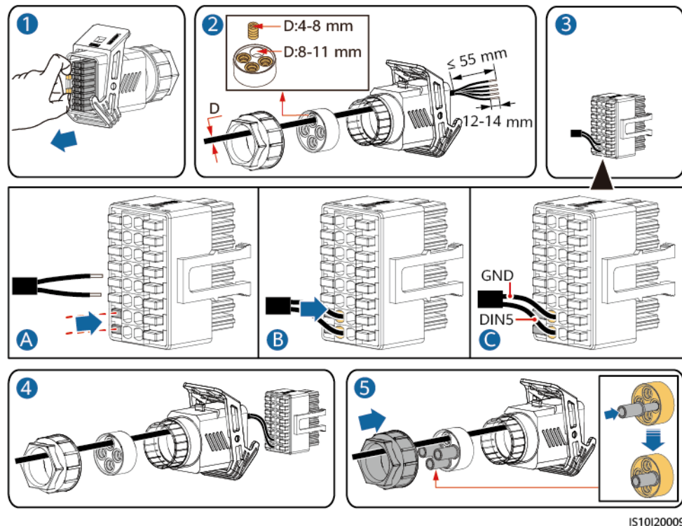
Abbildung 5-40 Kabelmontage
