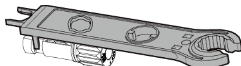
Abbildung 5-14 Entfernen eines DC-Steckverbinders
