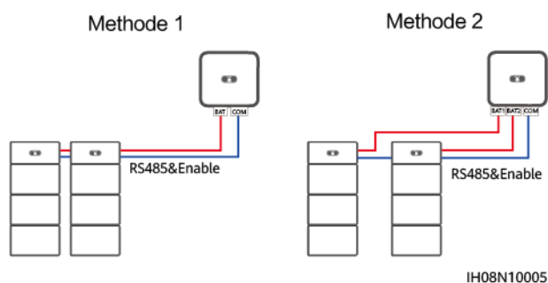
Abbildung 2-7 Anschluss des Wechselrichters an zwei Batterien
