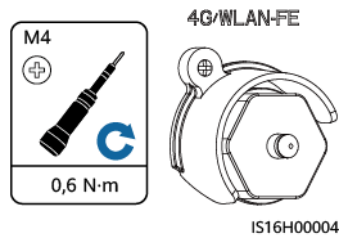
Abbildung 5-50 Installation der Anti-Diebstahl-Komponenten für den Smart Dongle
