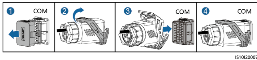
Abbildung 5-39 Sichern des Signalkabelsteckverbinders
