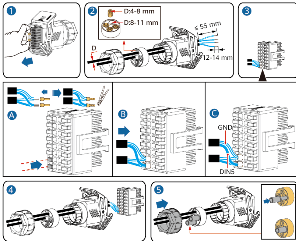
Abbildung 5-46 Installieren von Kabeln
