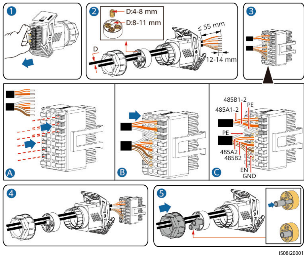
Abbildung 5-36 Installieren von Kabeln
