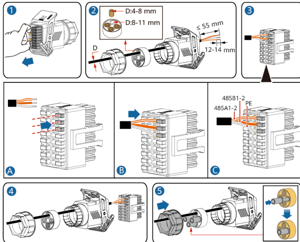
Abbildung 5-34 Kabelmontage
