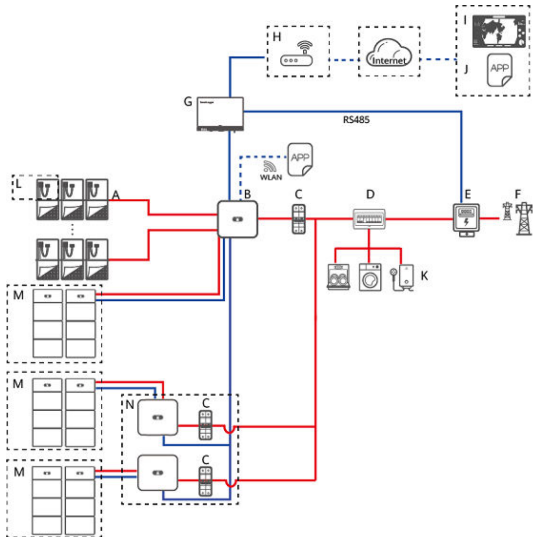
Abbildung 2-6 SmartLogger-Vernetzung (die Komponenten in den gestrichelten Kästen sind optional)
