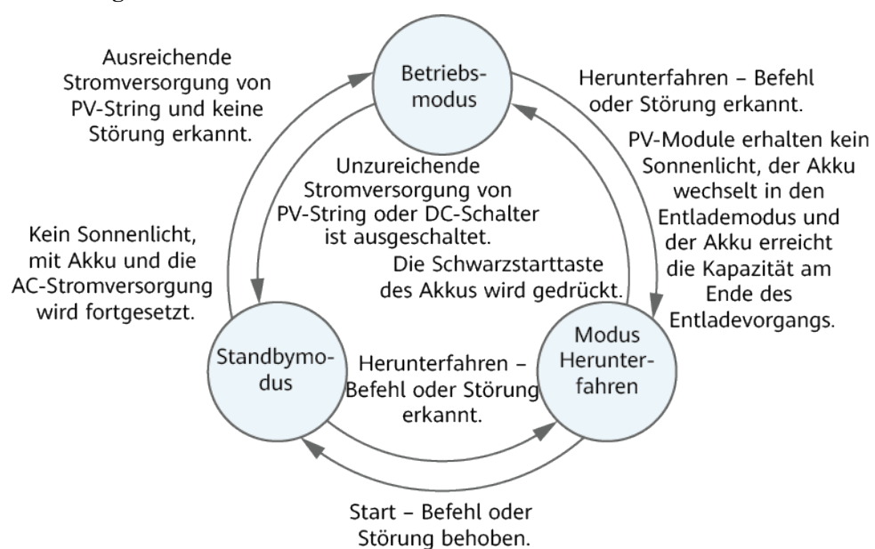
Abbildung 2-11 Arbeitsmodi
