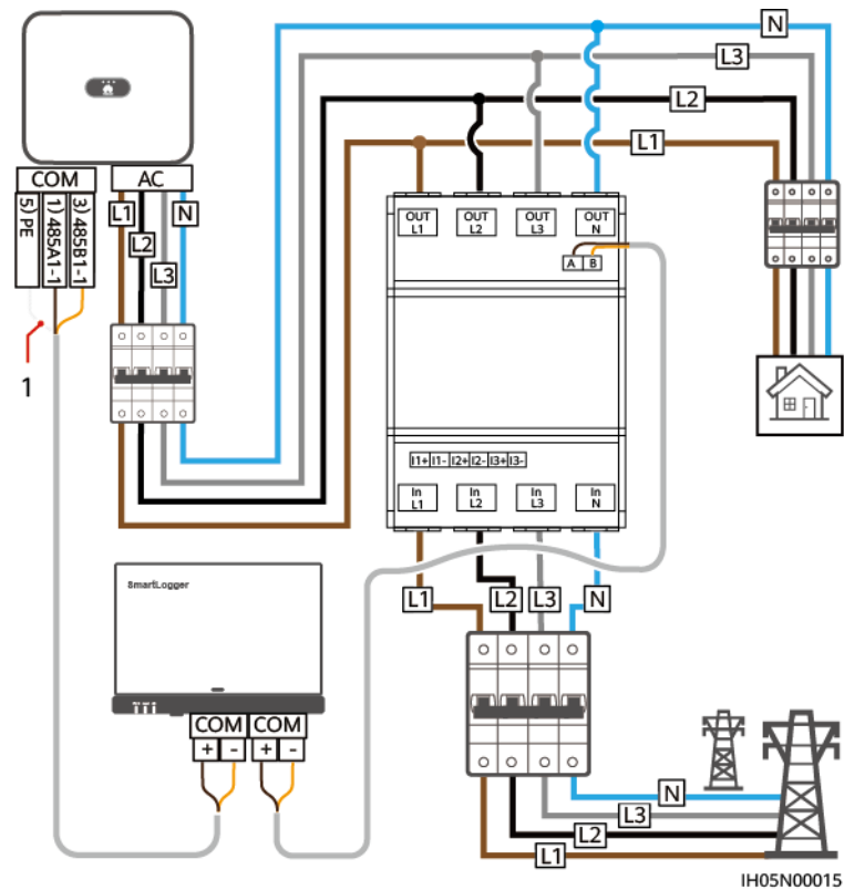
Abbildung 5-29 Dreiphasige vieradrige Direktverbindung (SmartLogger-Vernetzung)
