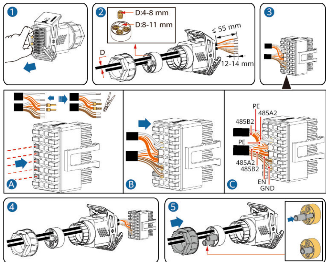
Abbildung 5-32 Installieren von Kabeln
