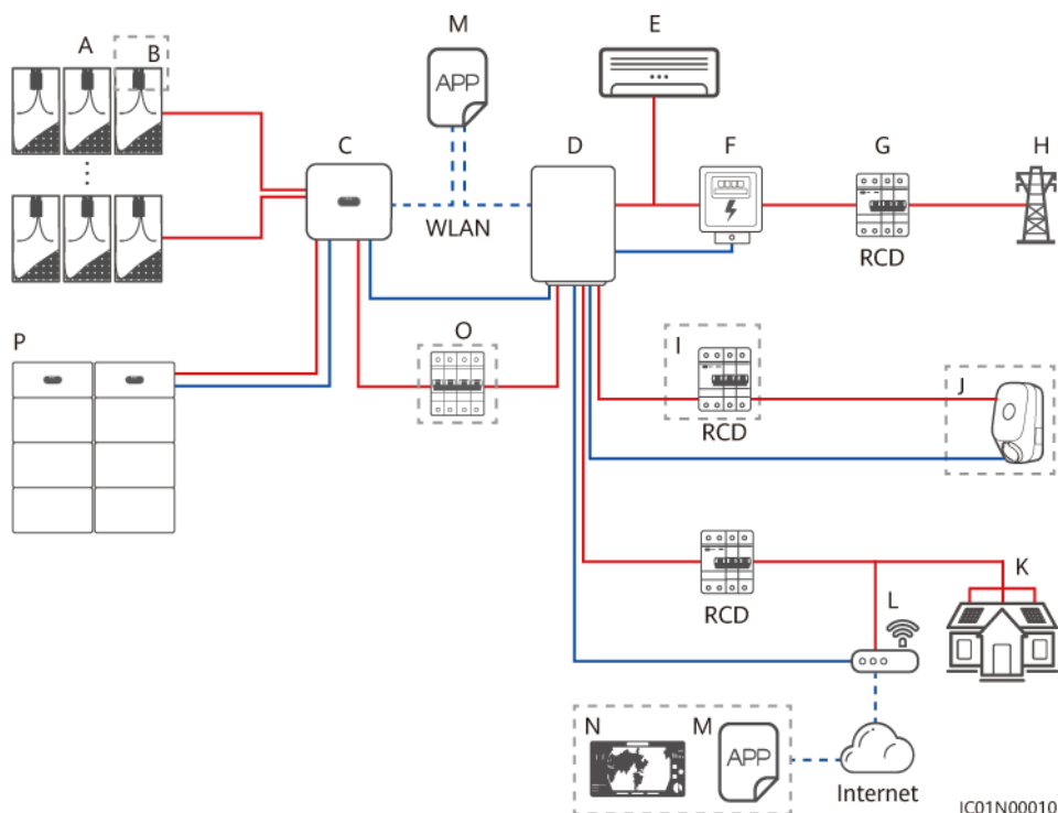
Abbildung 2-5 Vernetzung mit einigen an den SmartGuard angeschlossenen Lasten (die Komponenten in gestrichelten Kästchen sind optional)
