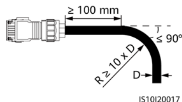
Abbildung 5-10 Verkabelungsanforderungen
