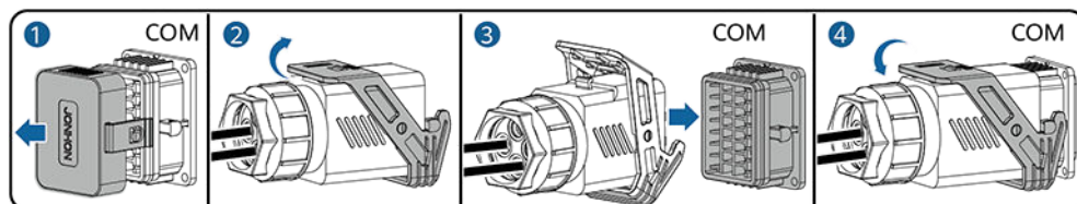
Abbildung 5-47 Sichern des Signalkabelsteckverbinders
