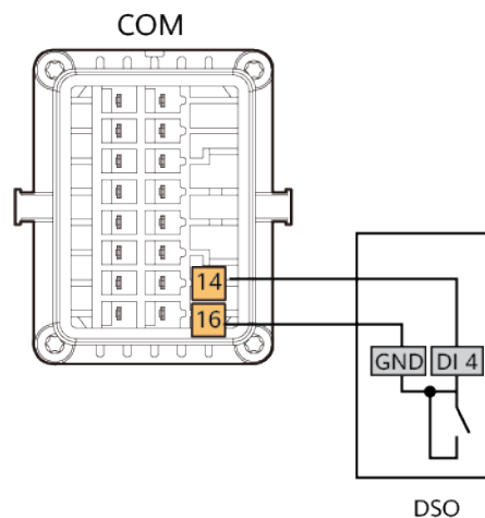
Abbildung 7-9 Kabelverbindungen
