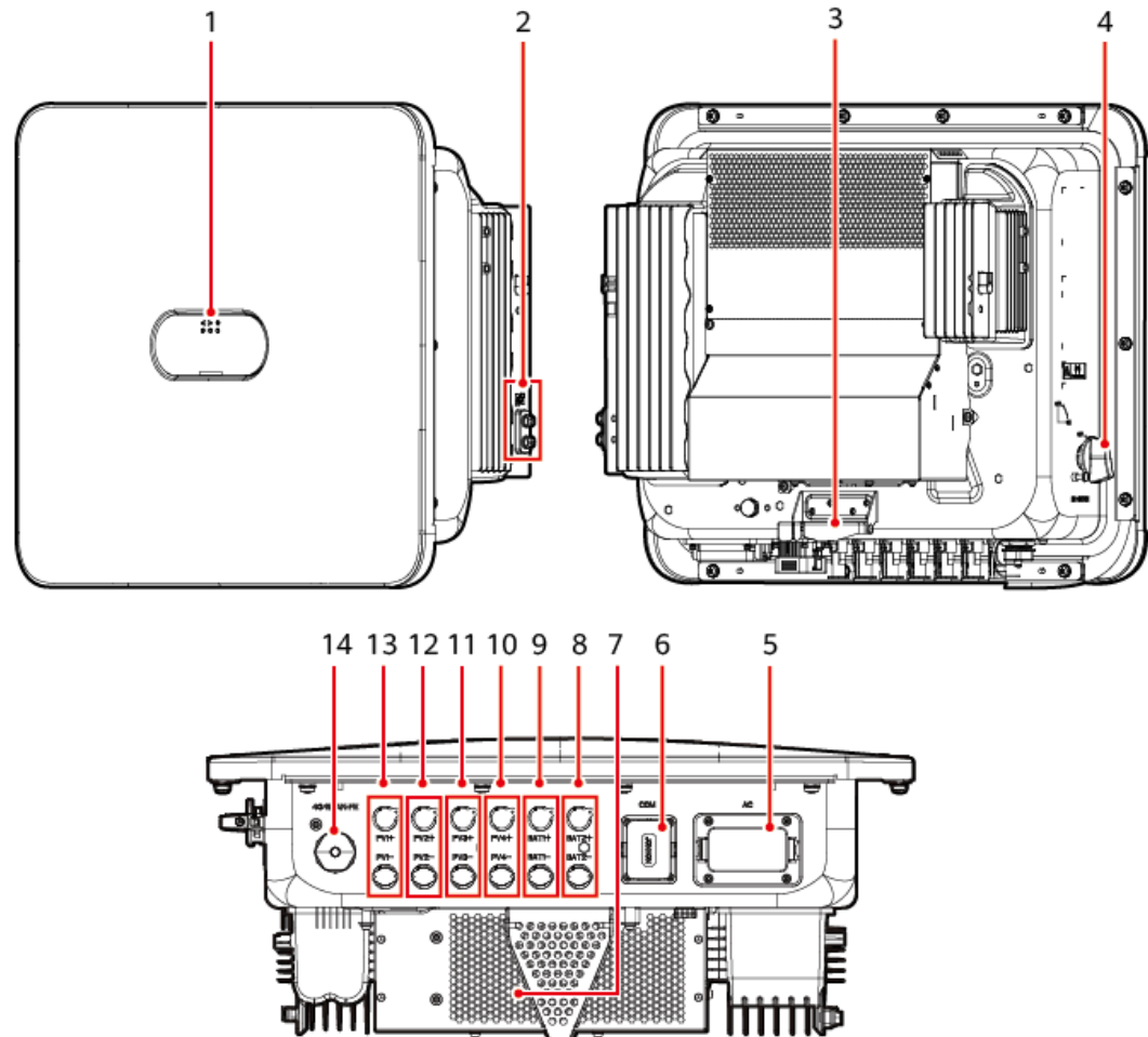
Abbildung 2-10 Aussehen
