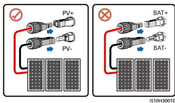
Abbildung 5-12 Verbindung
