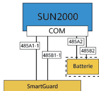
Abbildung 5-20 SmartGuard-Vernetzung (die Komponente im gestrichelten Kasten ist optional)
