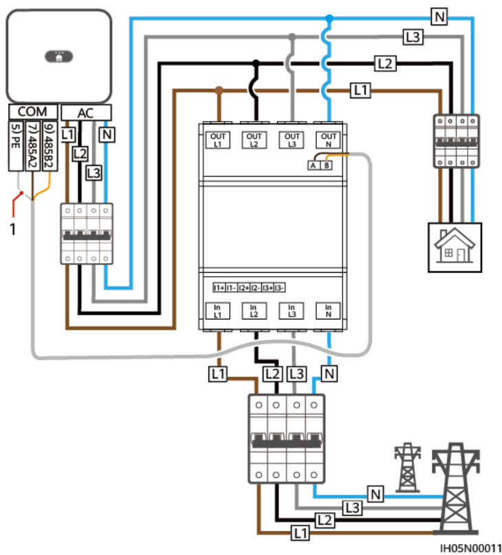
Abbildung 5-27 Dreiphasige vieradrige Direktverbindung (Smart Dongle-Vernetzung)
