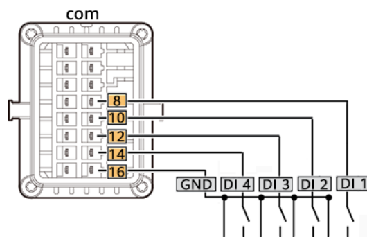
Abbildung 5-42 Kabelverbindung
