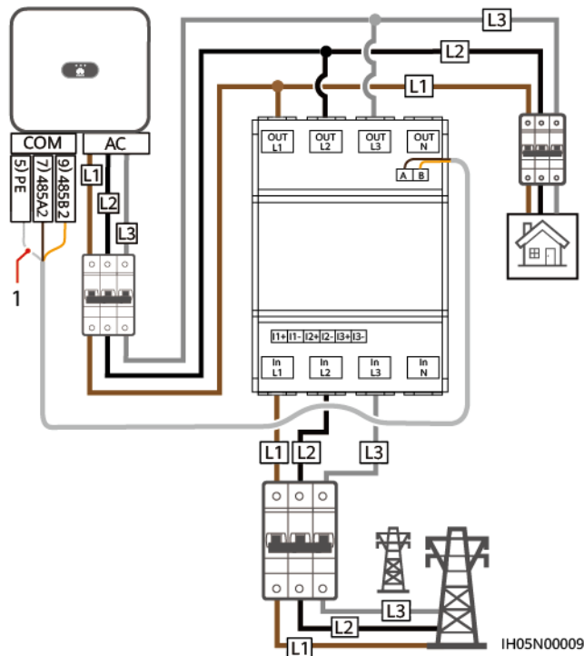
Abbildung 5-26 Dreiphasige dreiadrige Direktverbindung (Smart Dongle-Vernetzung)
