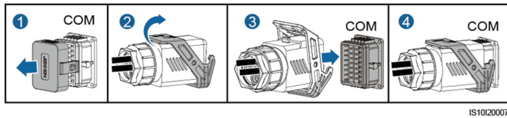
Abbildung 5-37 Sichern des Signalkabelsteckverbinders
