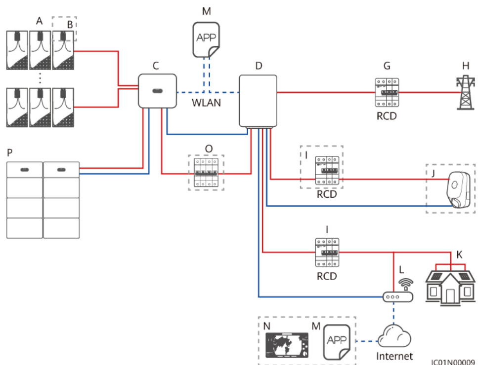
Abbildung 2-4 Vernetzung mit allen an den SmartGuard angeschlossenen Lasten (die Komponenten in gestrichelten Kästchen sind optional)
