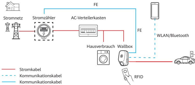
Abbildung2: Die Wallbox ist über den FE-Port mit dem Messgerät verbunden und nicht mit der Cloud-Plattform verbunden.
