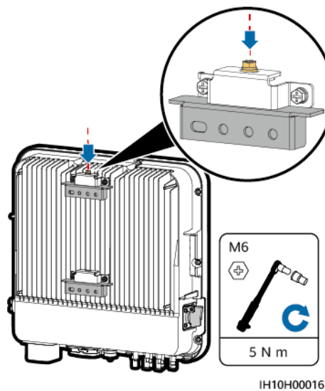
Abbildung 4-13 Montage des Wechselrichters
